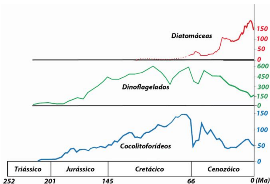
Figura 3.13. Evolução do número de espécies fitoplanctônicas durante o Mesozoico e o Cenozóico (ver tabela cronostatigráfica da Figura 1.1). No eixo horizontal, Ma= milhões de anos. No eixo vertical: número de espécies.
