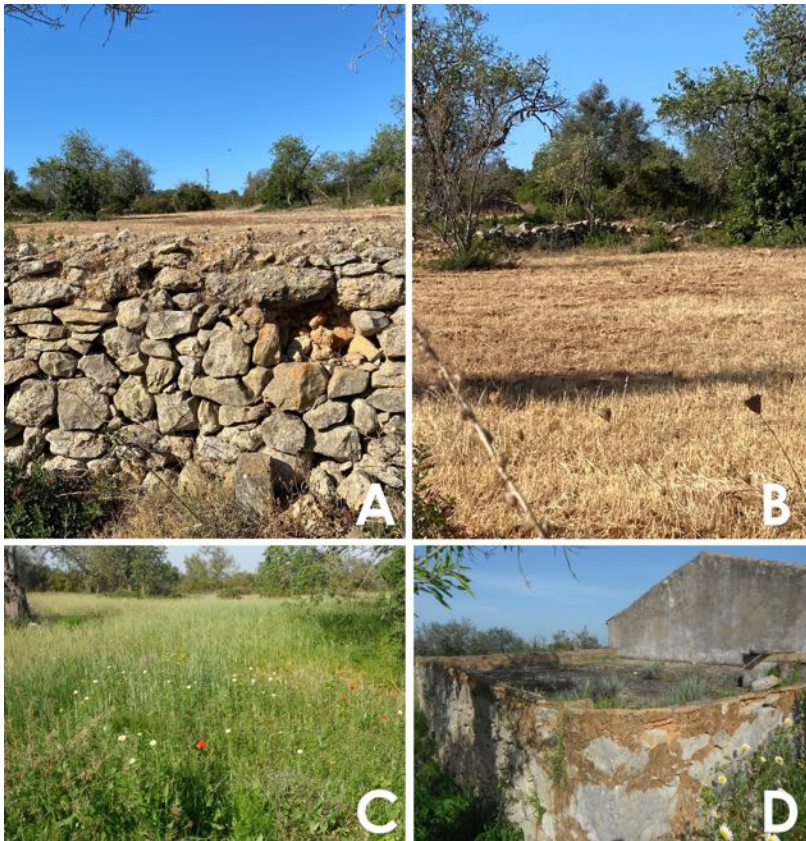
Figura 7.9. A e B: chãs (neste caso, aplanamentos cársicos) no Planalto do Escarpão. C: chã cultivada com cereais e D: casa com eira, adjacente ao campo da fotografia C. Na fotografia A, note o muro de suporte construído em pedra seca, que não constitui uma barreira ecológica.
