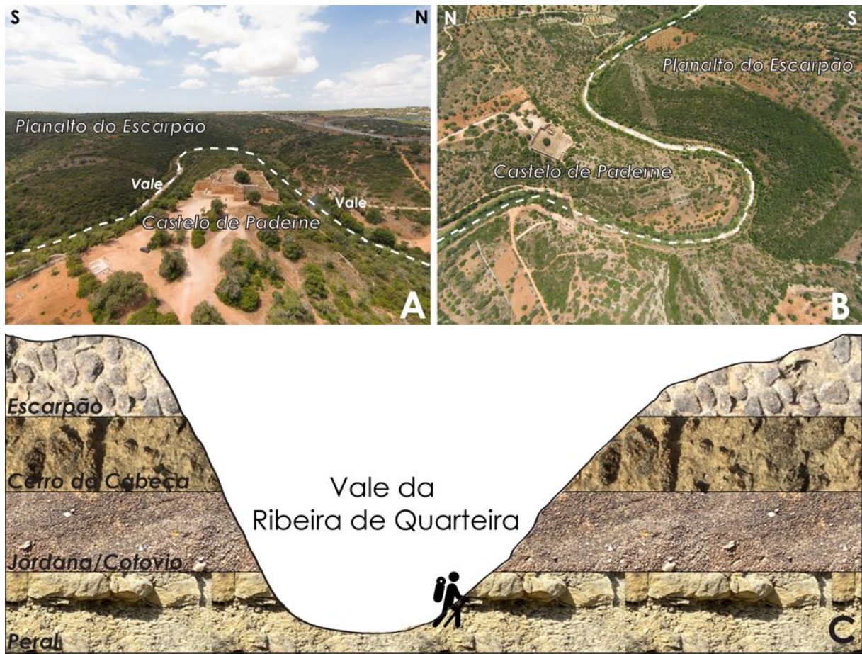
Figura 4.2. A e B: Fotografias do Planalto do Escarpão centradas no Castelo de Paderne abraçado pelo meandro (curva) da Ribeira de Quarteira. C: Esquema (sem escala) da estratigrafia das formações geológicas no Planalto do Escarpão e do modo como são intersectadas pelo vale da Ribeira de Quarteira.
