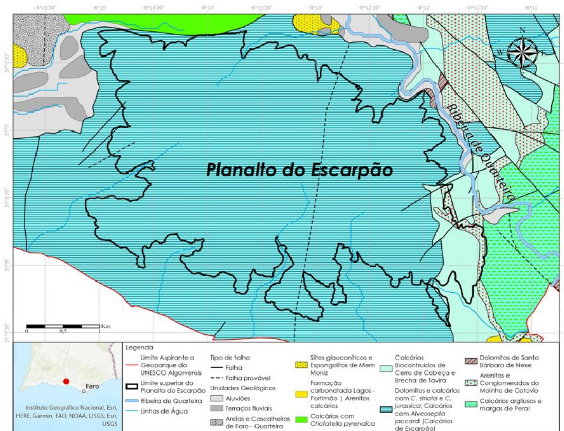
Figura 4.1. Localização e geologia do Planalto do Escarpão.
