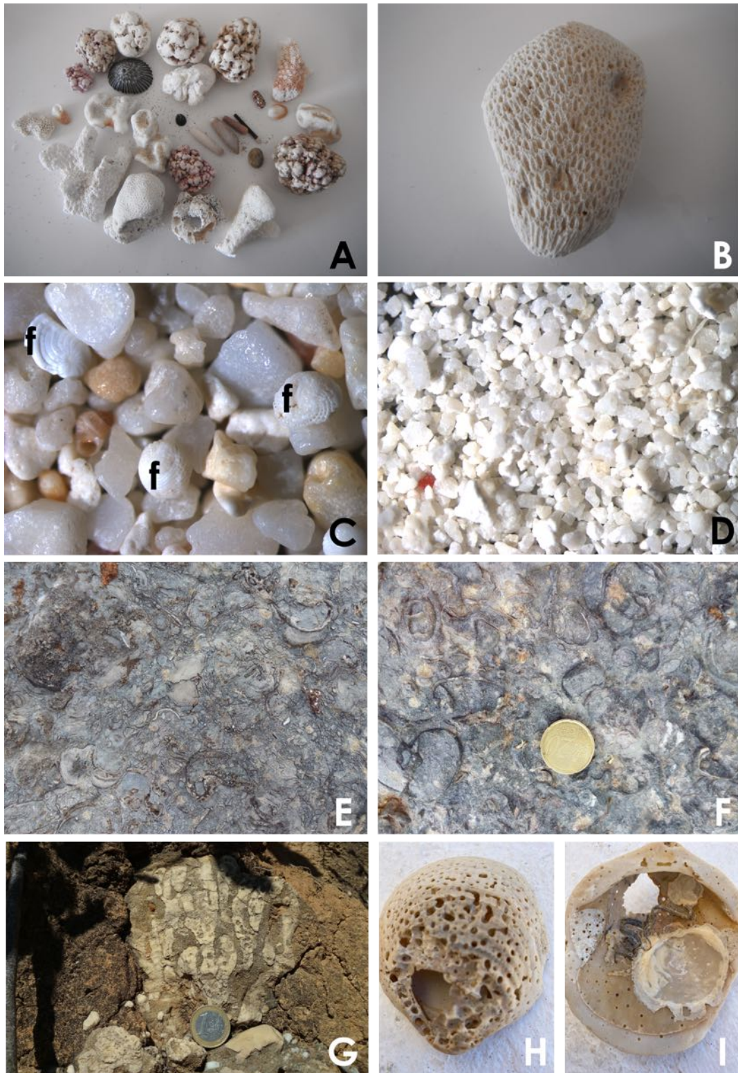
Figura 3.10 A: bioclastos recolhidos numa praia havaiana, resultantes da quebra do recife adjacente: fragmentos de diversas espécies de coral, gastrópodes e espículas de ouriço-do-mar; B: fragmento de coral; C: areia de uma praia em Cuba, constituída por grãos de quartzo e bioclastos (f-foraminíferos); D: areia de uma praia nas Maldivas, inteiramente bioclástica; E e F: brecha recifal, com fragmentos de estromatoporóides, esponjas e rudistas (Formação de Escarpão); G: fósil de coral (Formação de Escarpão); H: concha de bivalve atual intensamente bioperfurada facilitando a sua quebra; I: face ventral da mesma concha que em H, mostrando que serviu de substrato para a fixação de outros organismos. Por este motivo, a identificação dos fósseis nem sempre é fácil.
