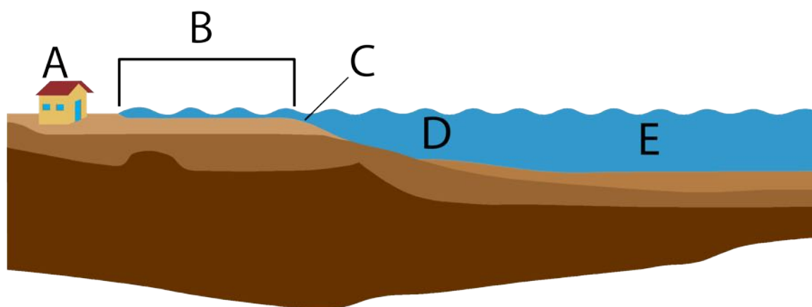
Figura 3.2. Esquema de uma margem continental, composta por plataforma continental (B), talude continental (C) e elevação continental (D), entre os domínios costeiro (A) e marinho profundo (E), com os quais estabelece trocas de massa e de energia. Ver secção 3.2 para explicações adicionais.
